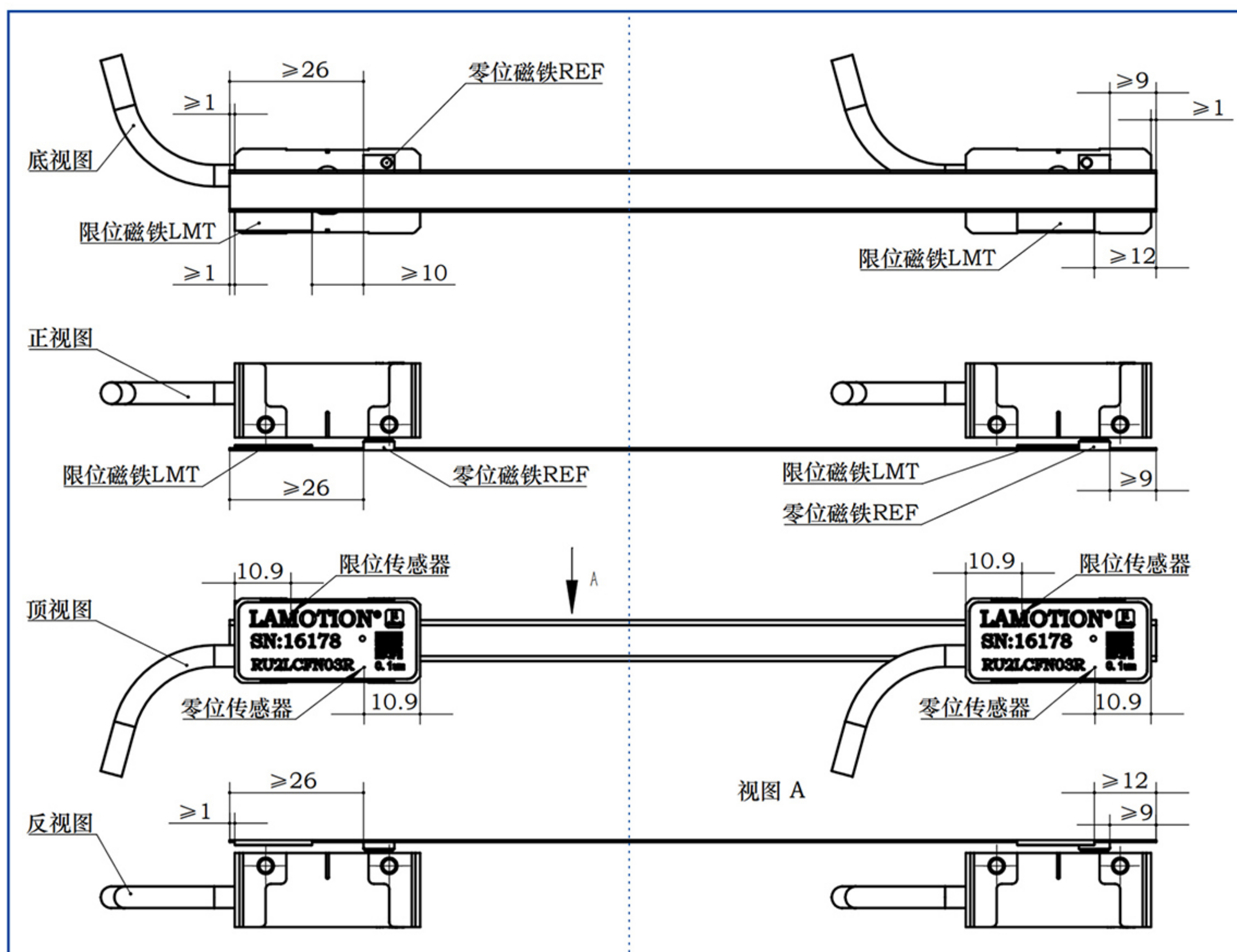
栅尺左端安装零位磁铁
