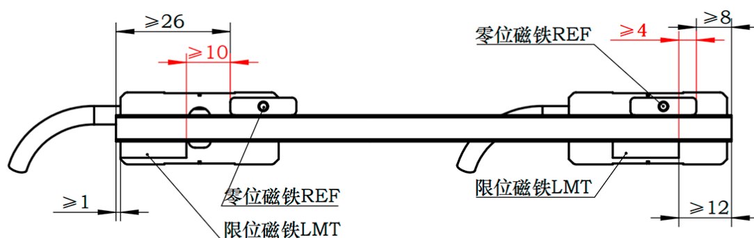
栅尺左端安装零位磁铁
