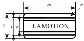
端压片 D2-ET
