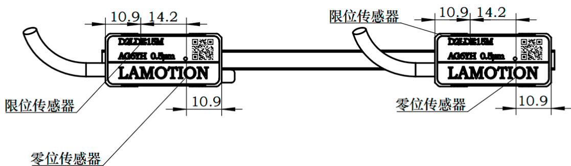
俯视图
