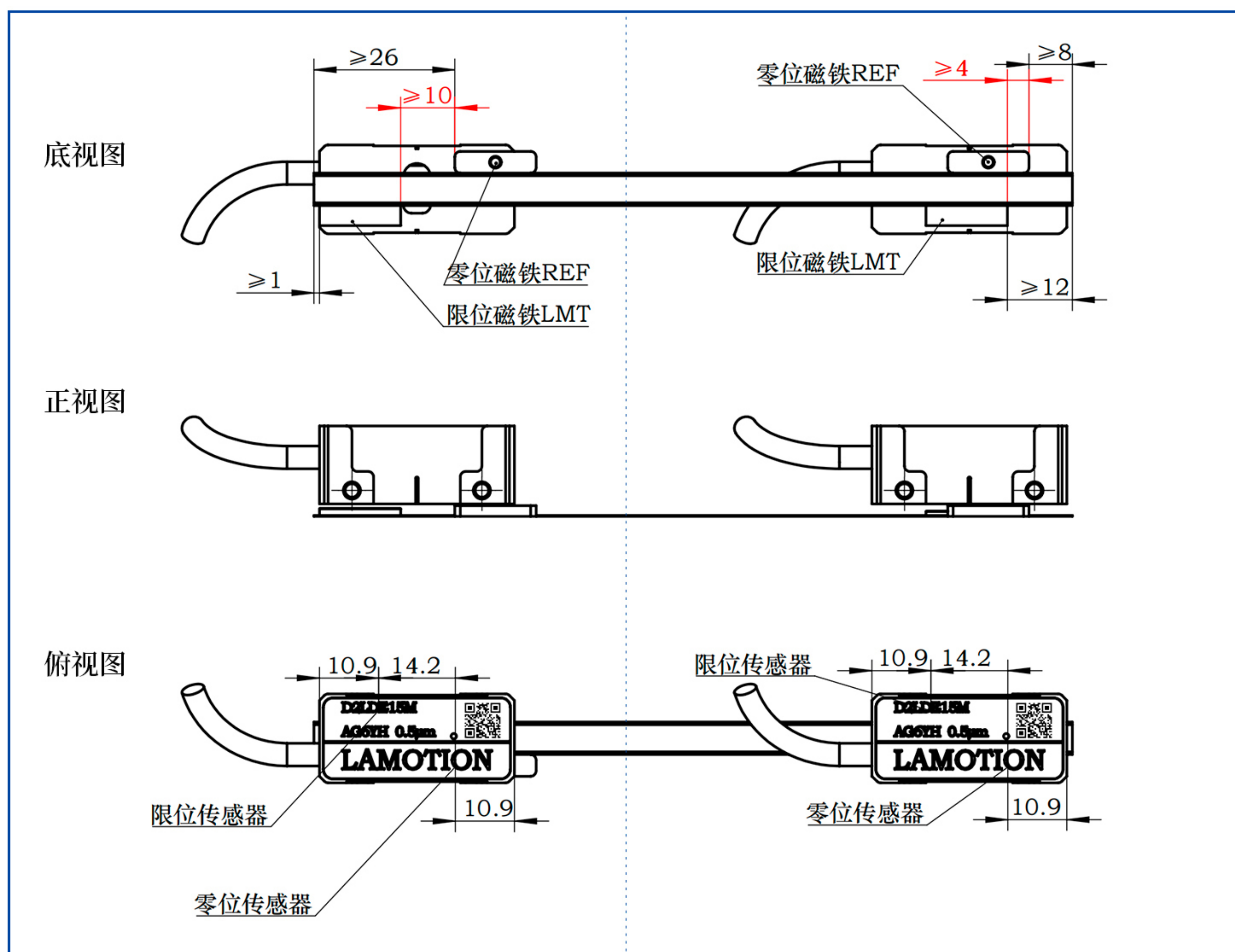
栅尺左侧安装零位磁铁
