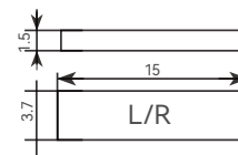
左限位磁铁 RX2-LMT-L-15 右限位磁铁 RX2-LMT-R-15
